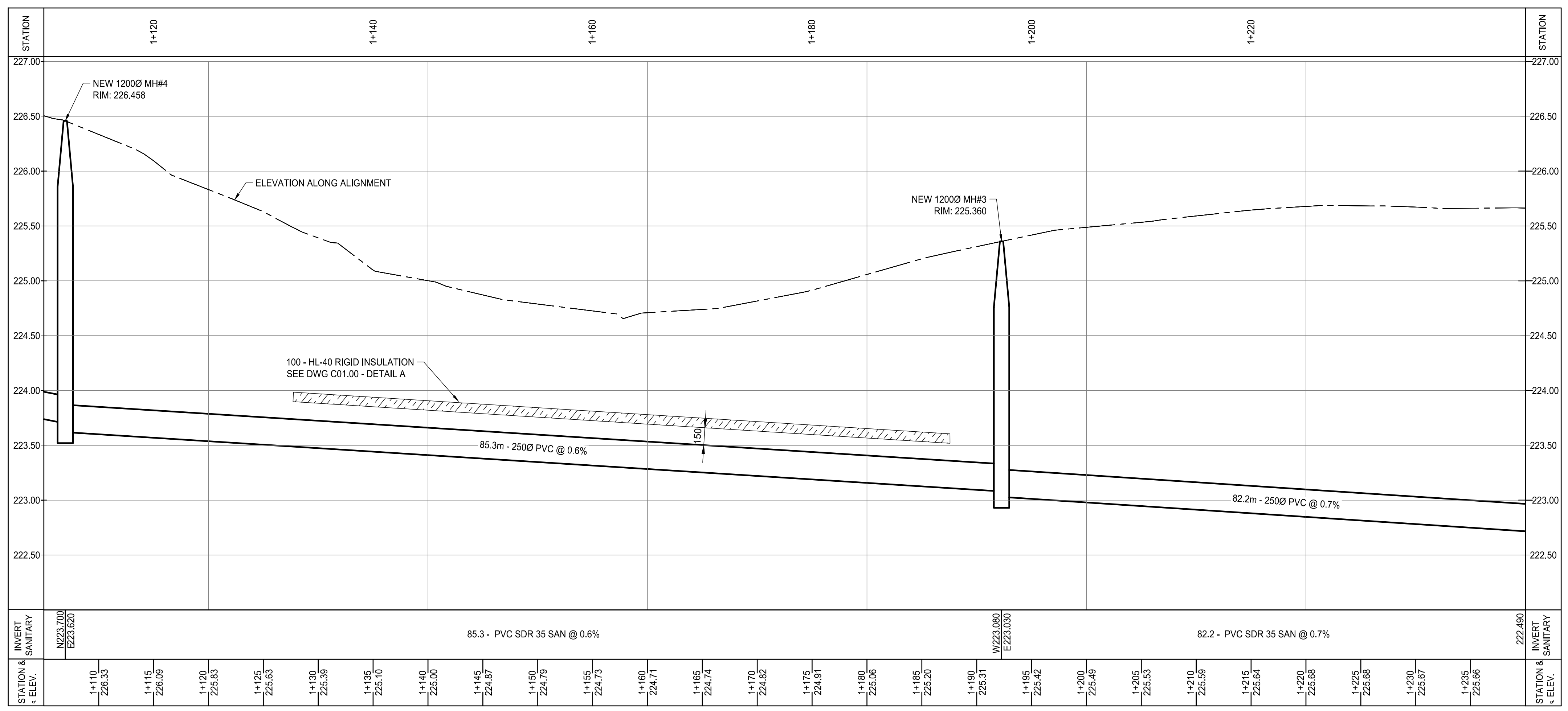
PROFILE STA 1+105 TO 1+240 SCALE: H:1:250 V:1:25
