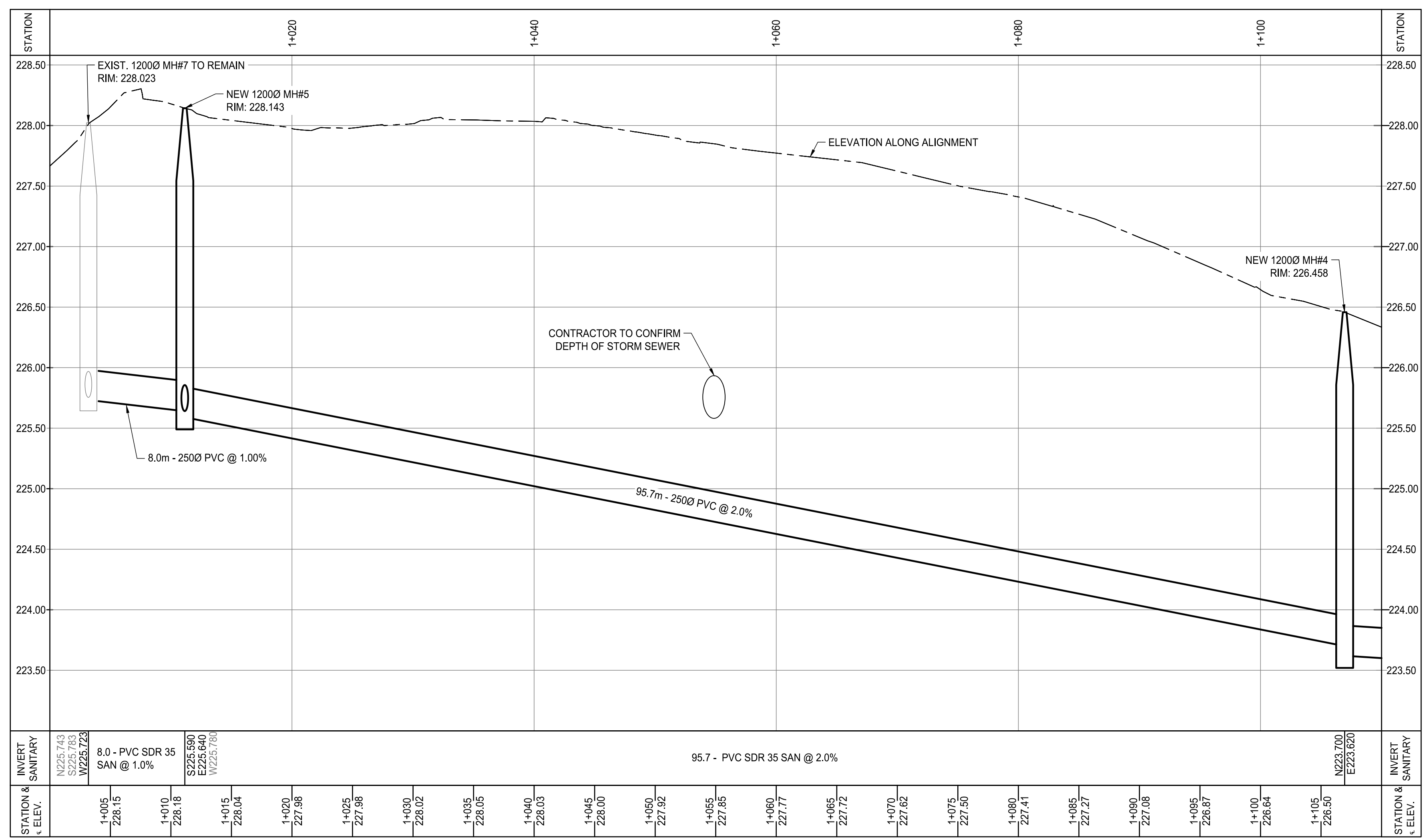
PROFILE STA 1+000 TO 1+110 SCALE: H:1:250 V:1:25
