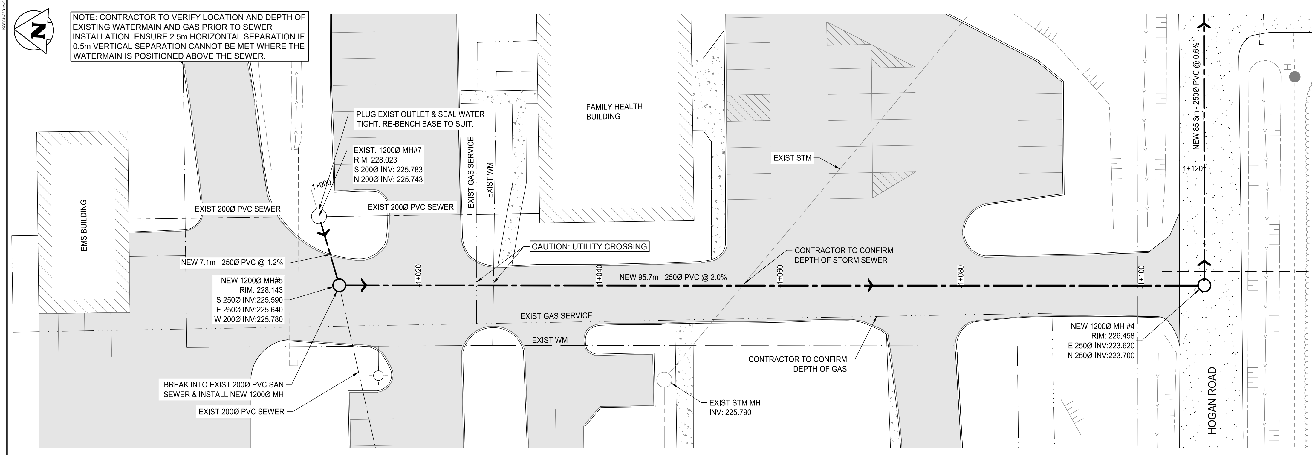
PLAN VIEW STA 1+000 TO 1+110 SCALE: 1:250
